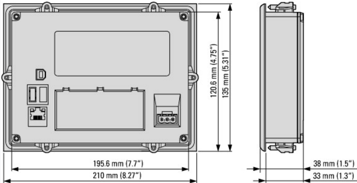
Dimensions
